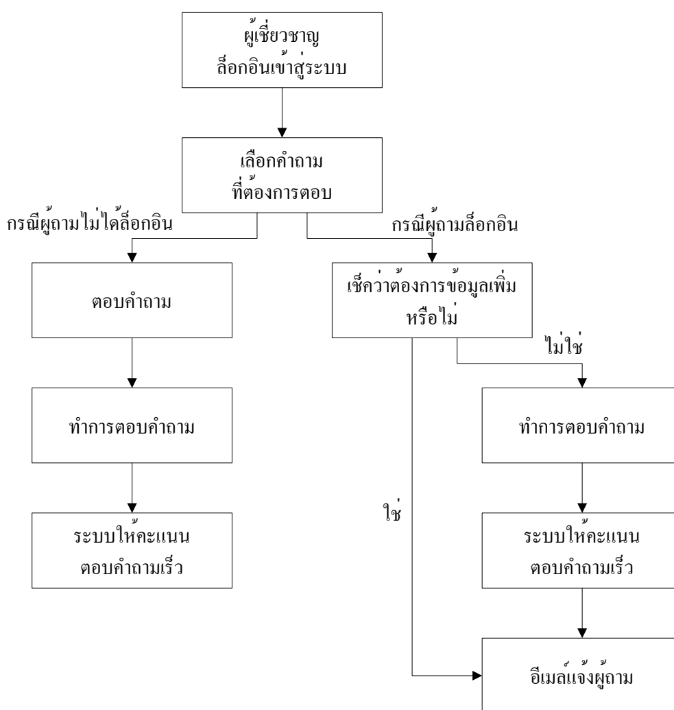
รูปที่ 3-94 แสดงโฟลว์ชาร์ตของฟังก์ชันการตอบคำถาม
