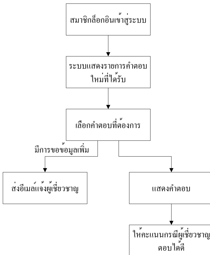
รูปที่ 3-100 แสดงโฟลว์ชาร์ตของฟังก์ชันการดูคำถาม-คำตอบที่ตนถามกรณีเป็นสมาชิก
