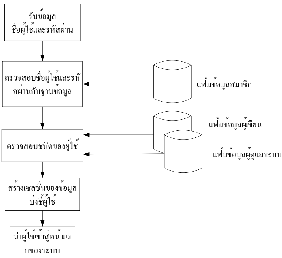
รูปที่ 3-9 แสดงหลักการทำงานของระบบการเข้าสู่ระบบ
