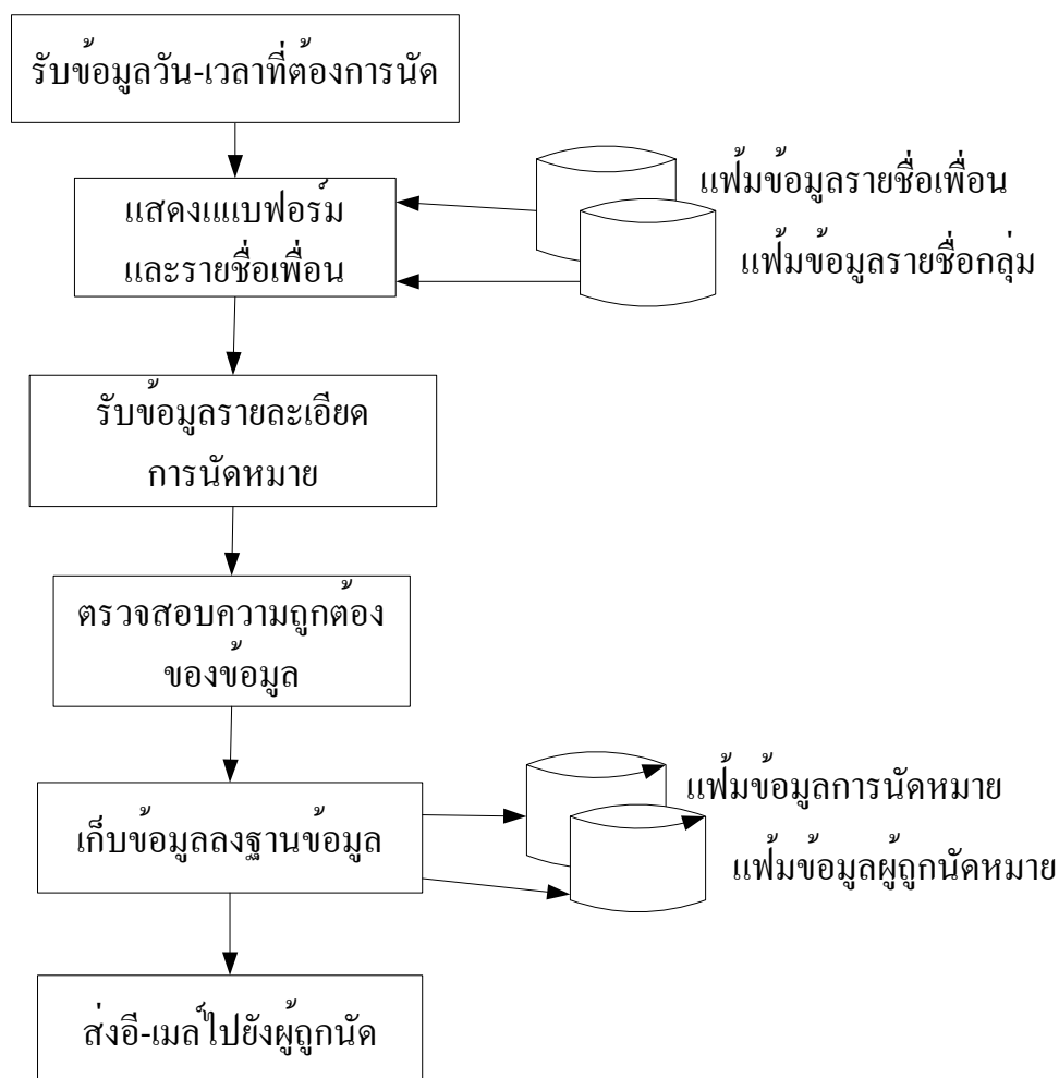
รูปที่ 3-61 แสดงหลักการทำงานของกรนัดหมายรายบุคคล
