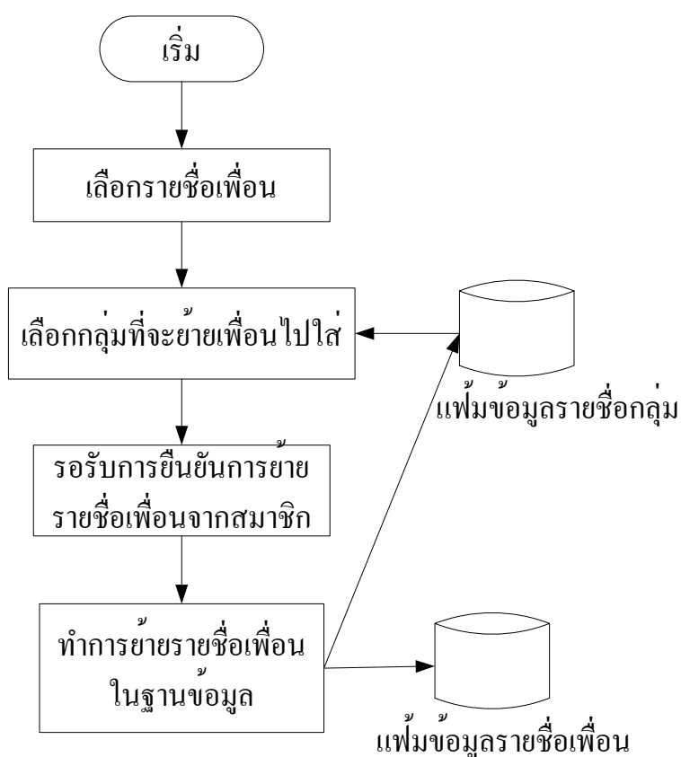
รูปที่ 3-28 แสดงหลักการทำงานย้ายรายชื่อเพื่อน
