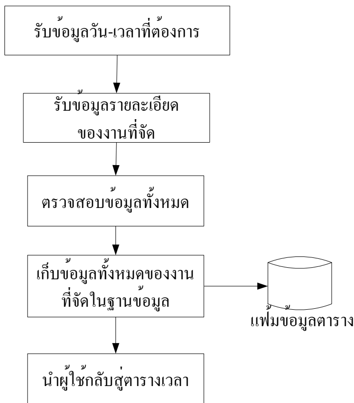
รูปที่ 3-49 แสดงหลักการทำงานของการจัดตารางเวลา
