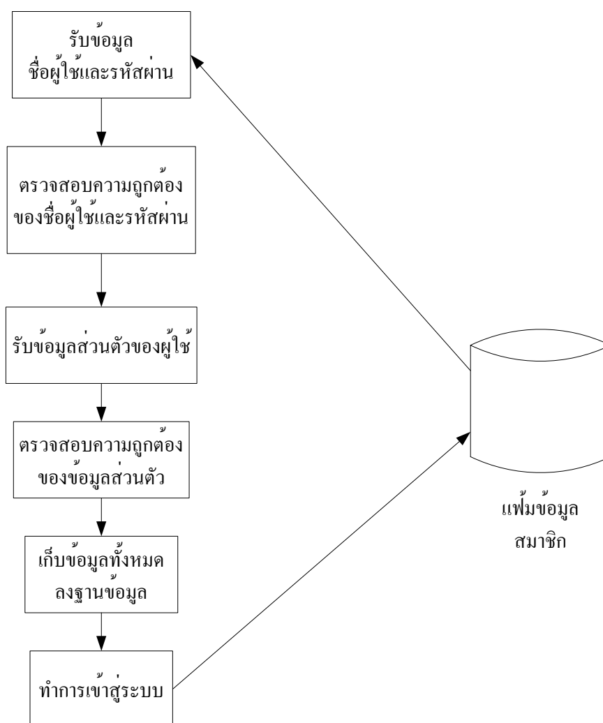
รูปที่ 3-4 แสดงหลักการทำงานของ การสมัครสมาชิก
