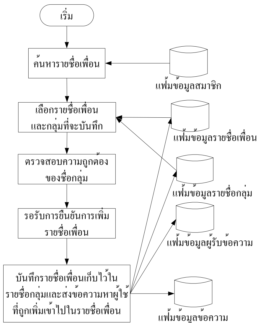
รูปที่ 3-21 แสดงหลักการทำงานในการเพิ่มรายชื่อเพื่อน
